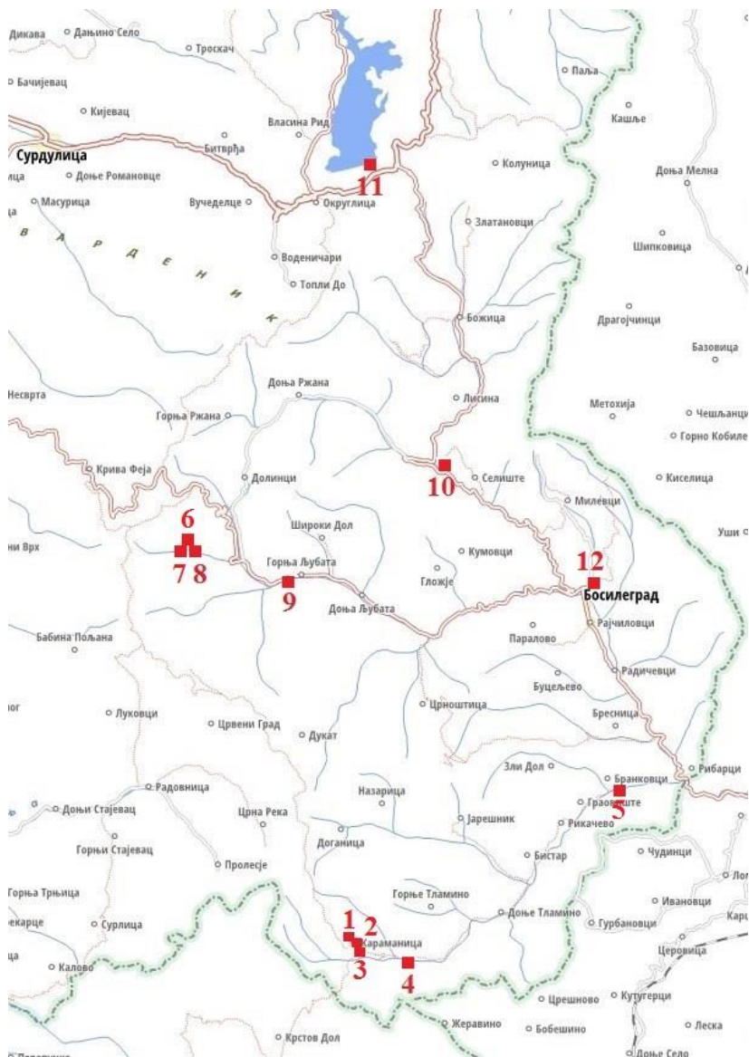
Скица на Босилеградско краиште и местата от които са взимани водните проби.
